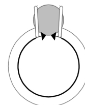
Circonferenza
